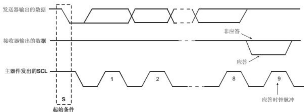
图7 I²C总线的应答
