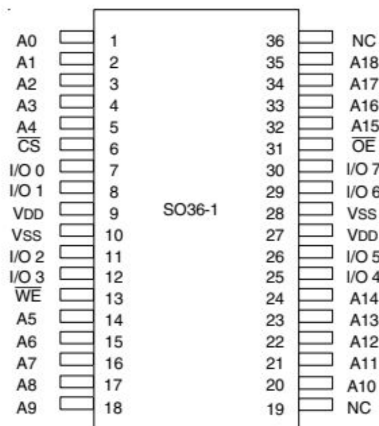
SOJ Top View
