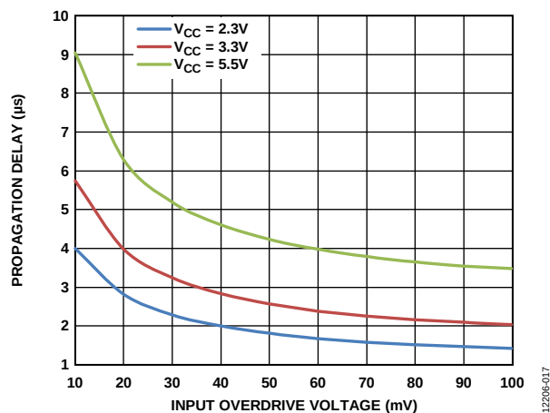
图17. 传播延迟与输入过驱电压的关系(高到低)
