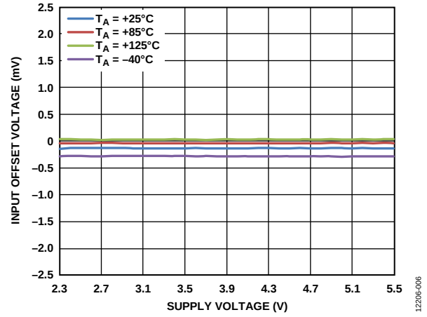
图6. 不同温度下输入失调电压( V_{OS} )与电源电压( V_{CC} )的关系( V_{CM} = 1\text{ V} )
