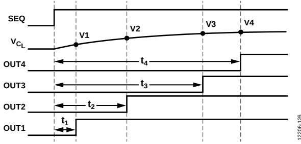
图26. 可编程时序控制电路时序图
