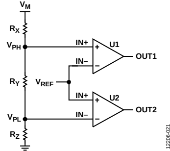
图22. 正欠压/过压监控配置
