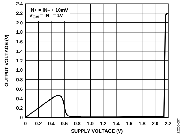
图7. 输出电压( V_{OUT} )与电源电压( V_{CC} )的关系( R_{PULLUP} = 10\text{ k}\Omega )
