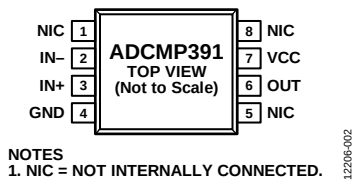
图2. 引脚配置
