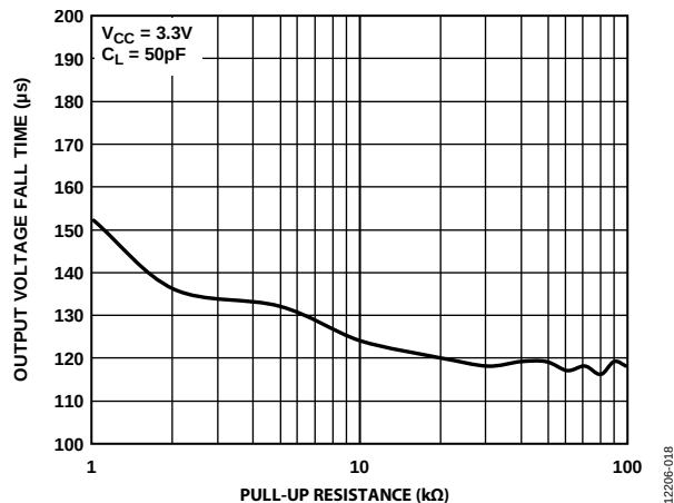
图18. 输出电压下降时间( t_f )与上拉电阻( R_{PULLUP} )的关系
