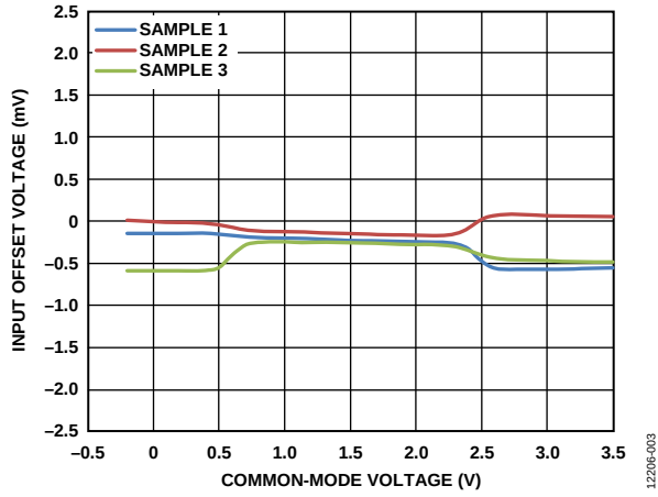
图3. 输入失调电压( V_{OS} )与共模电压( V_{CM} )的关系( V_{CC} = 3.3\text{ V} )
