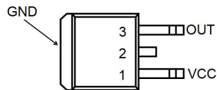
TO-263-3
