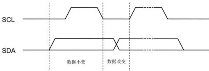
图8 数据转变
