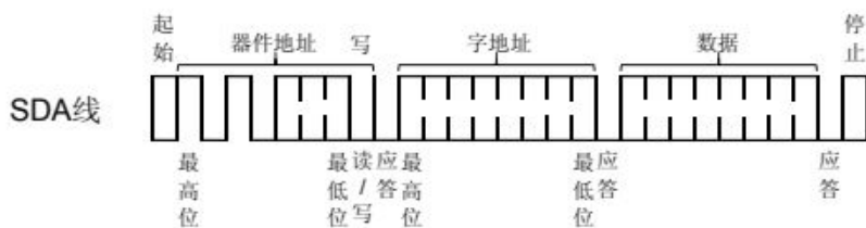
图11 字节写
