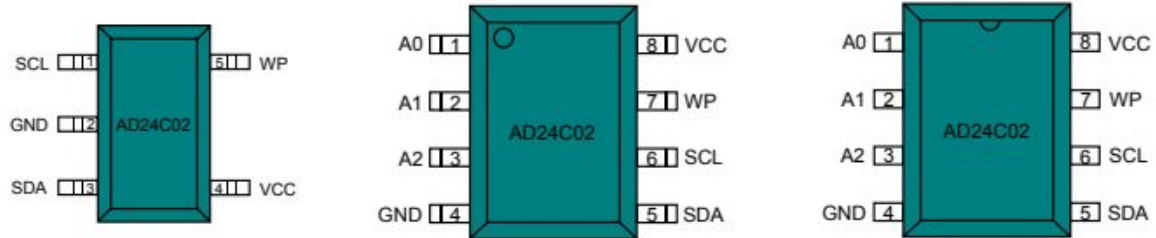
图2 AD24C02引脚定义图
