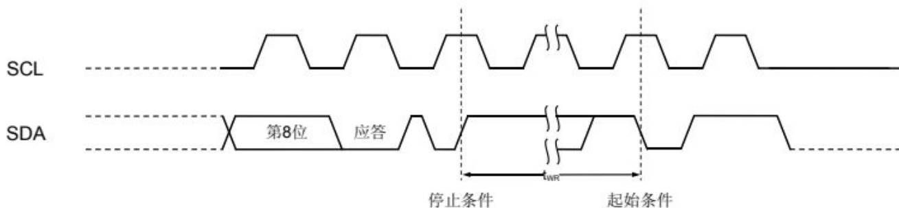
图5 总线时序
