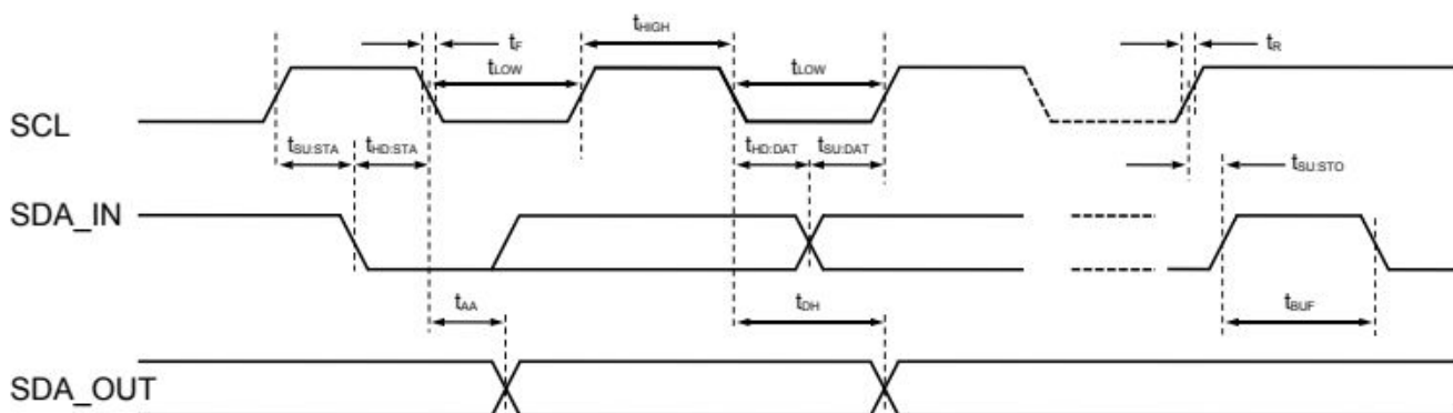
图5 总线时序
