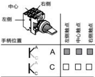
触点状态, 2位置
