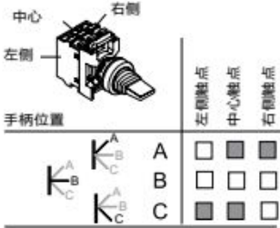
触点状态, 3位置
