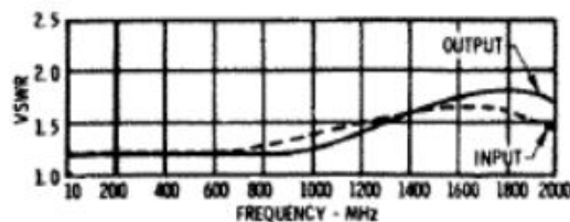
VSWR
