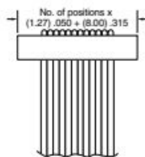
Strain Relief (-SR)
