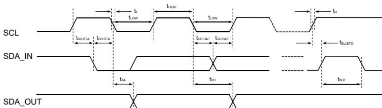
图5 总线时序
