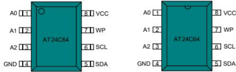
图2 AT24C64引脚定义图
