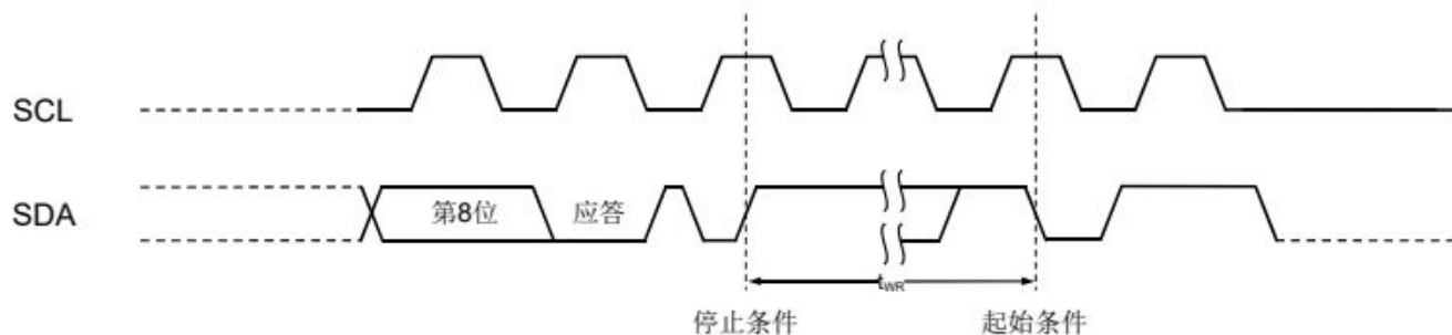
图5 总线时序
