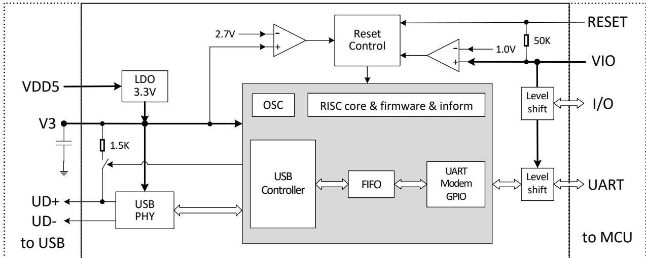
图 5-1 内部结构
