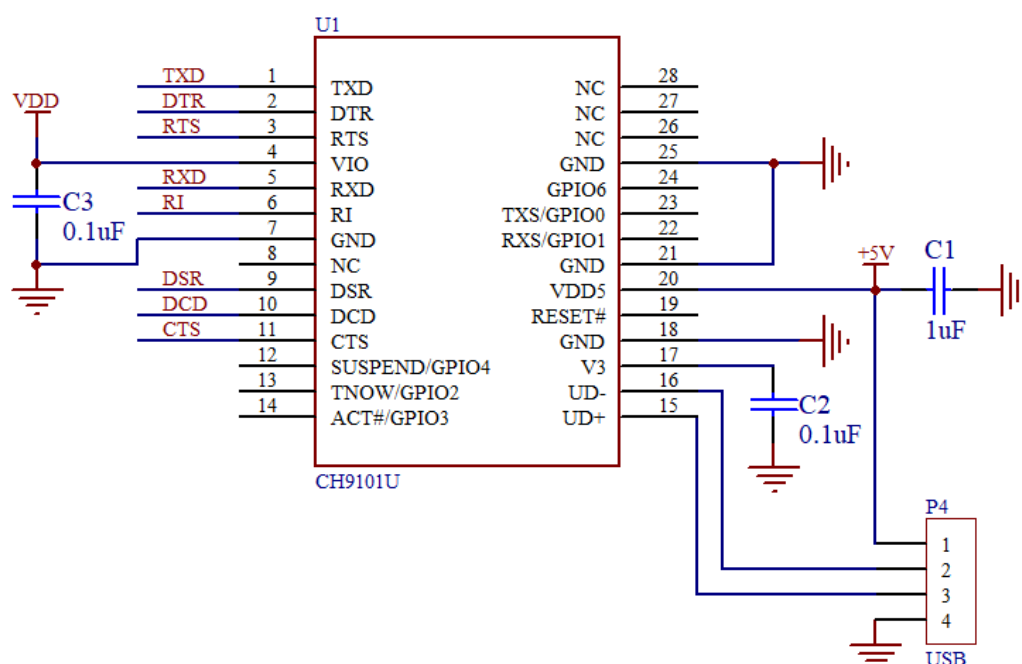
图 8-1 USB 转 9 线 TTL 串口的参考电路图
